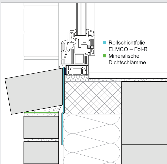
Einbauschnitt Fensterbrüstung zweischaliges Mauerwerk mit Abdichtung; Variante Folie in der Schalenfuge
