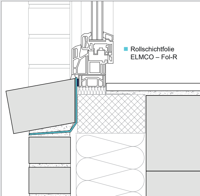
Einbauschritt Fensterbrüstung zweischaliges Mauerwerk mit Abdichtung; Variante Folie im Mörtelbett
