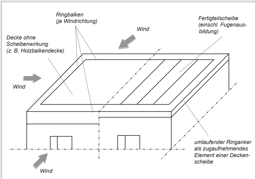
Bild 1: Wirkungsweise Ringanker/ Ringbalken
