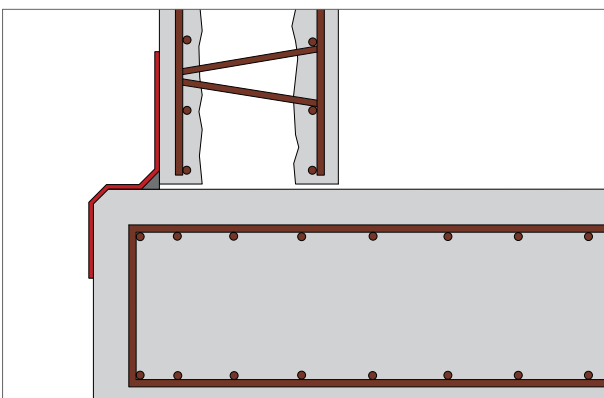
Abdichtung von horizontalen Arbeitsfugen im Anschlussbereich zwischen Sohle und Wand
