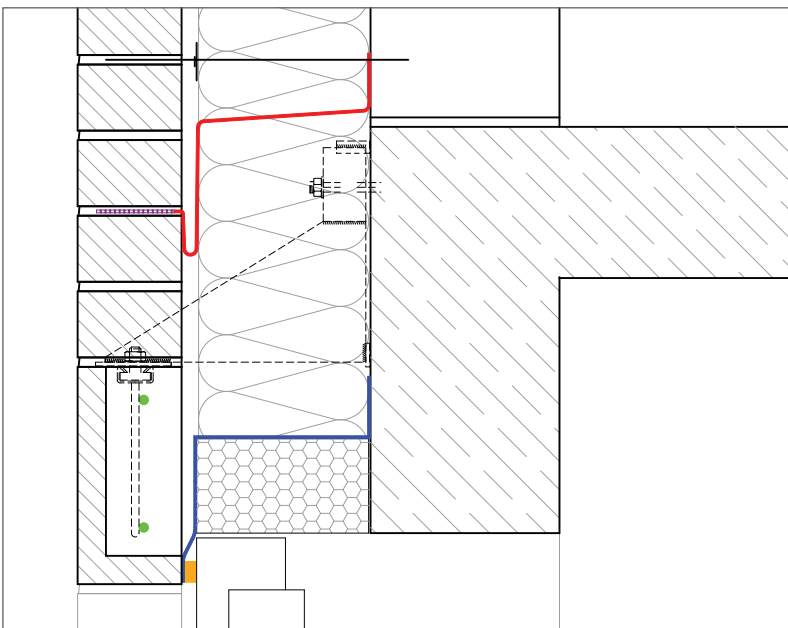
Lage der ELMCO – Fol als Sturzdrainage in Verbindung mit Fertigteilstürzen an Konsolkernen
