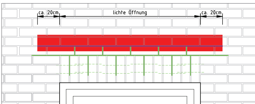
Lage der ELMCO – Fol als Sturzdrainage in Verbindung mit der Sturzbewehrung ELMCO – Ripp
